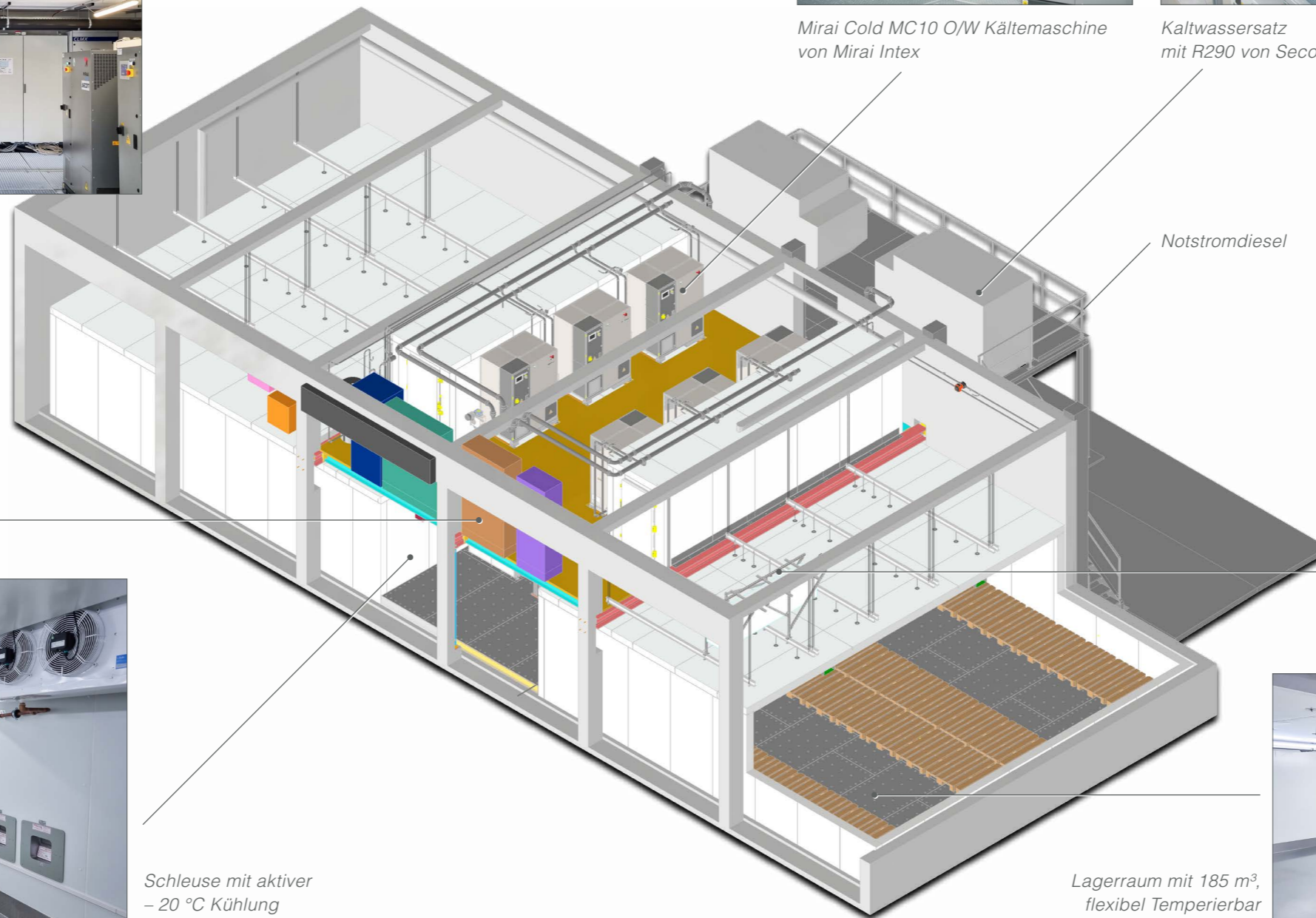
Maschinenraumkonditionierung
